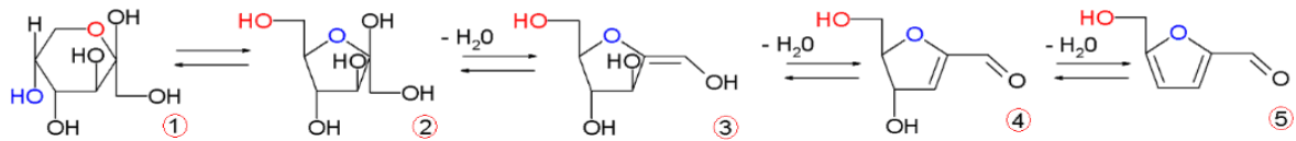
Figuur 2: van glucose naar hydroxymethylfural (Bron: wikipedia)
